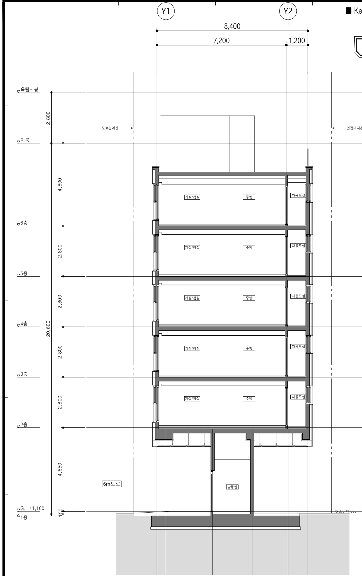
1 101동 대지형단면도 축척=1/120
