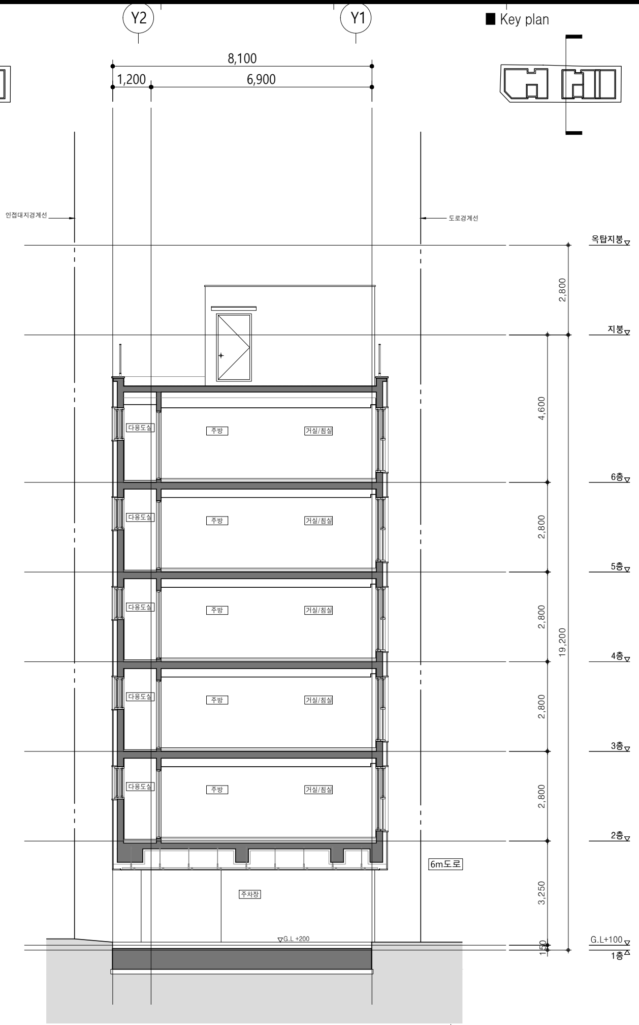
A 102동 대지형단면도 축척=1/120
