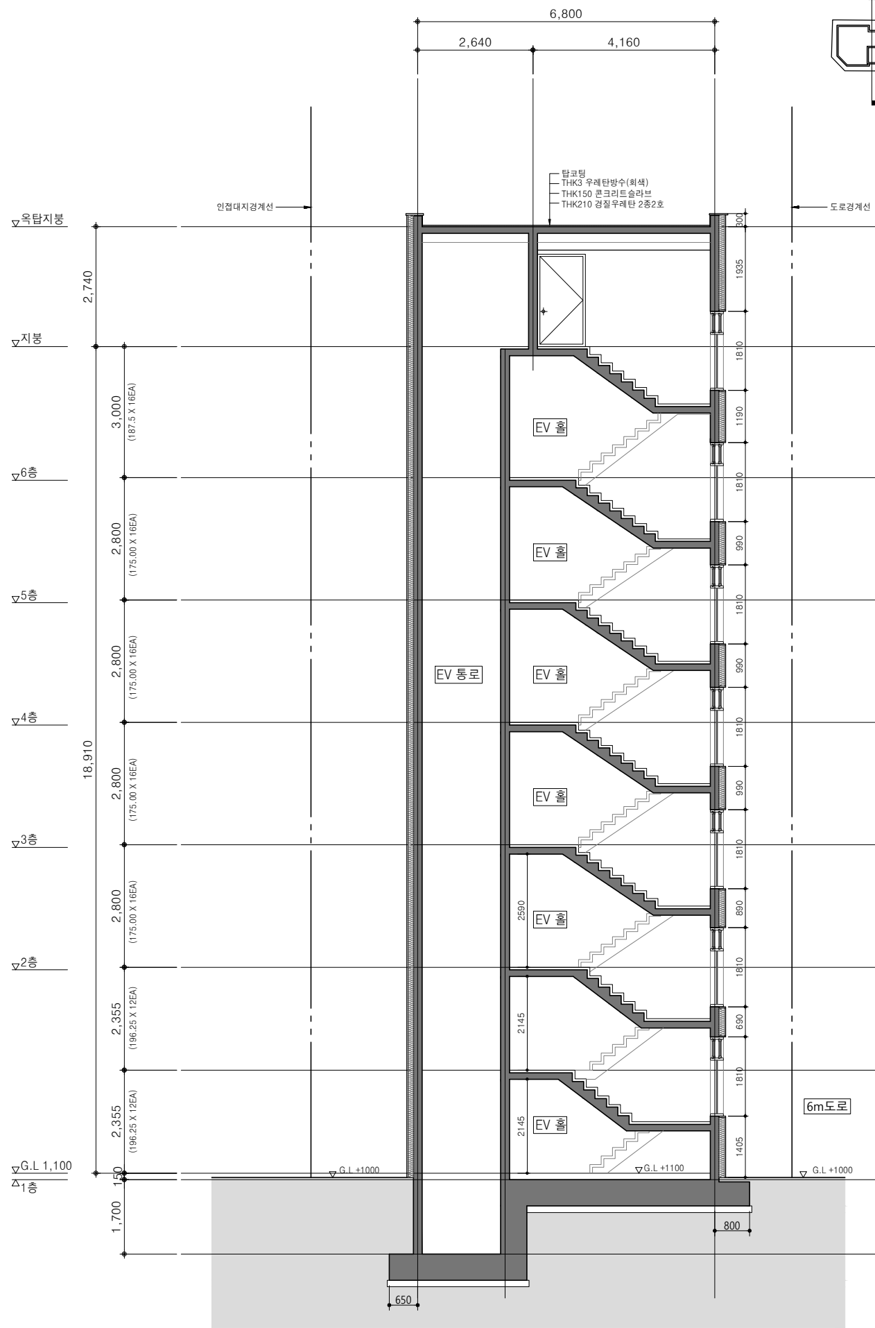
101동 계단단면도
