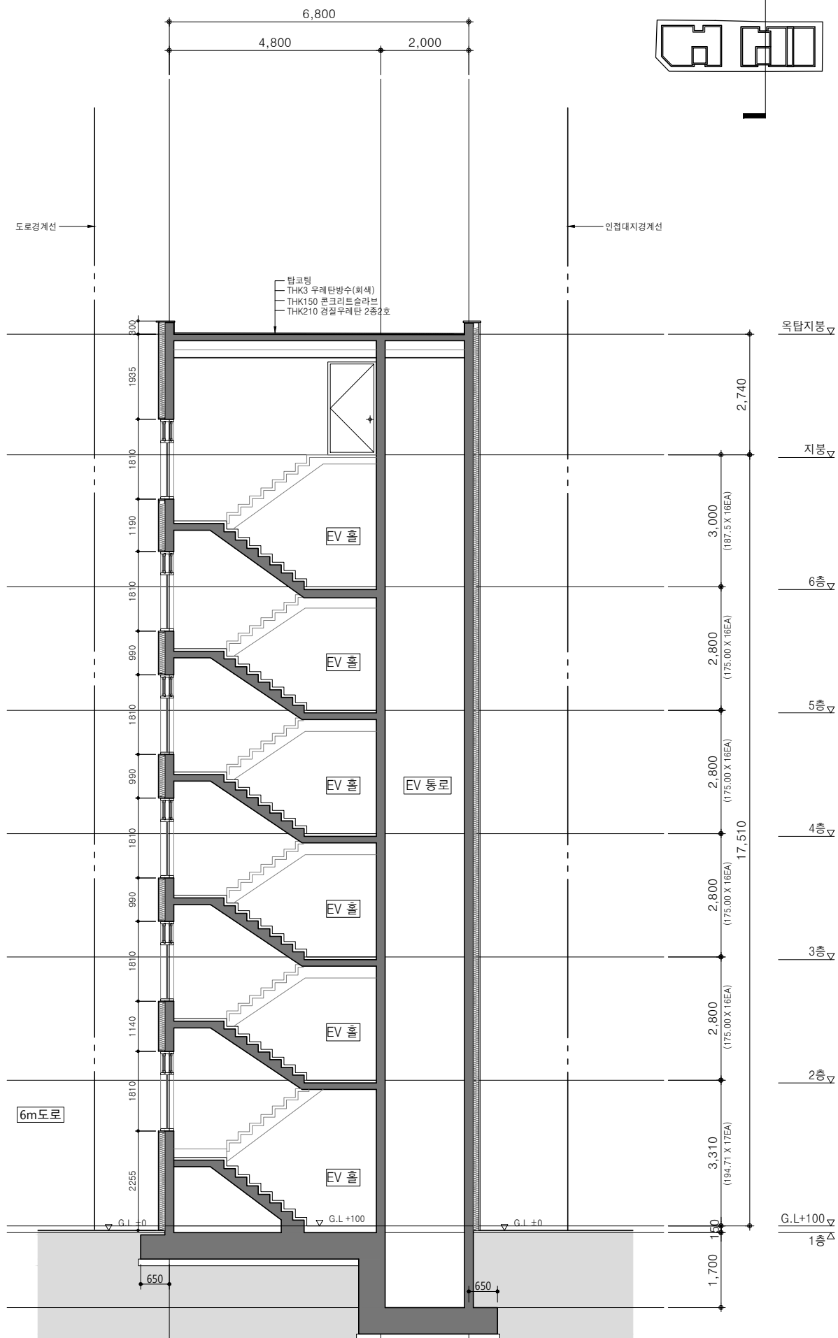
102동 계단단면도
